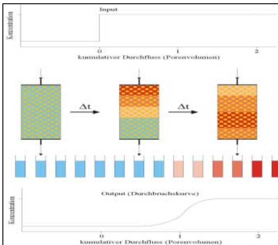
Abb. 11: Prinzip einer Durchbruchkurve (verändert nach GISI 1990)
