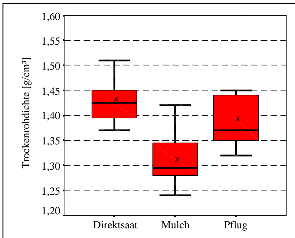
Abb. 15: Trockenrohddichte der Bodensäulen
