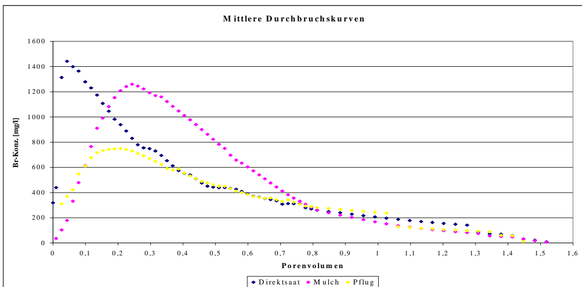
Abb. 20 Beregnungsversuch: Mittlere Durchbruchkurven
