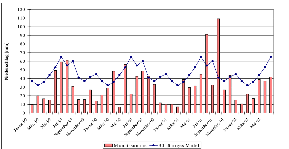
Abb. 6: Niederschlagsgang an der Klimamessstation Spröda (Leipziger Land) von Januar 1999 bis Juni 2002
