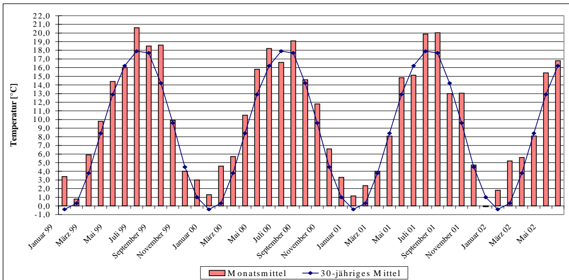
Abb. 5: Temperaturgang an der Klimamessstation Spröda (Leipziger Land) von Januar 1999 bis Juni 2002
