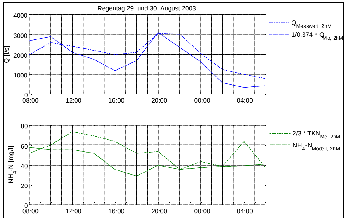
Abbildung 86: Vergleich des Ablaufs des ADL-Modells mit Zulaufsmesswerten der Kläranlage 2h-Mittelwerte 29. und 30.08.2003
