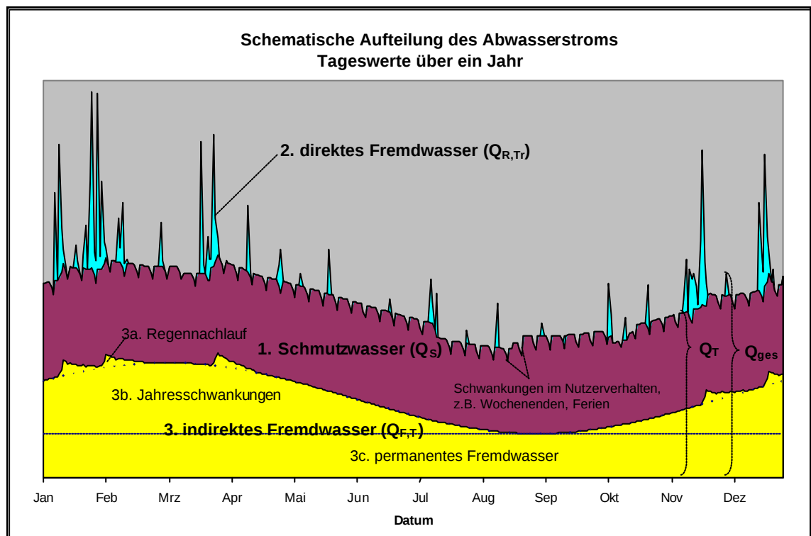
Abbildung 80: Schematische Aufteilung des Abwasserstroms
