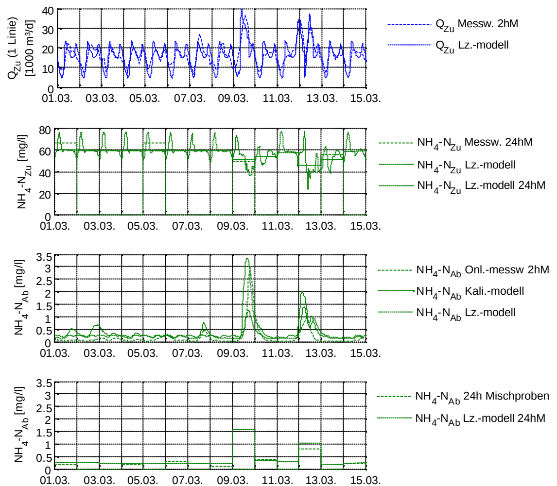
Abbildung 88: Ergebnis der Kalibrierung der Kläranlage für Ammonium
