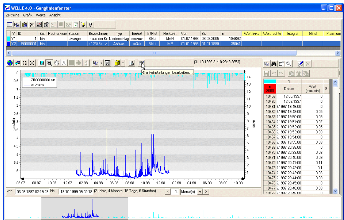
Abbildung 54: WELLE-Ganglinienfenster mit Niederschlags- und Abflusszeitreihe
