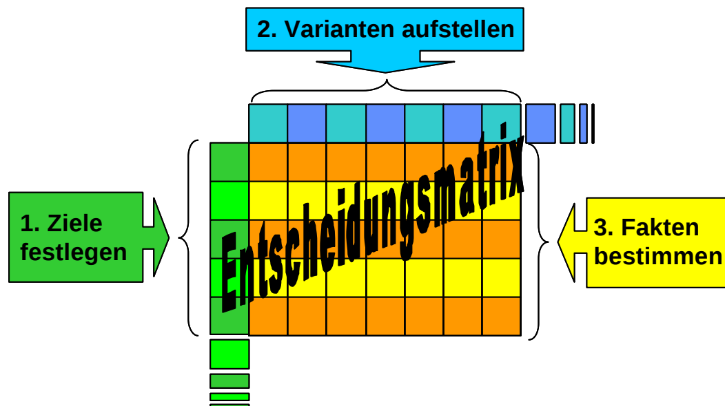
Abbildung 11: Entscheidungsmatrix (Prinzip)
