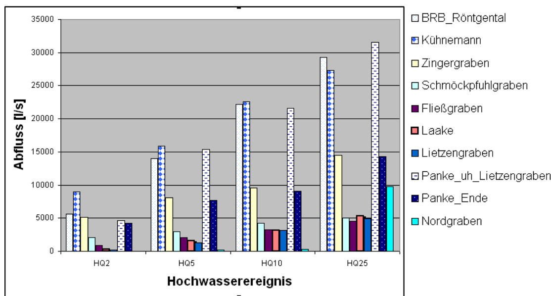
Abbildung 78: Hochwasserstatistik Ist-Zustand (31 Jahre RS Wedding)
