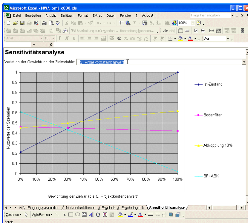
Abbildung 69: Excel-Bewertungstool – Sensitivitätsanalyse
