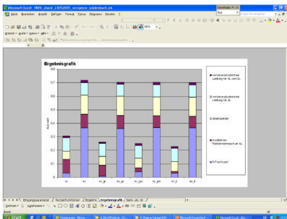
Abbildung 118: Die Nutzwerte der einzelnen Szenarien (Erläuterung der Abkürzungen s. Tabelle 29)
