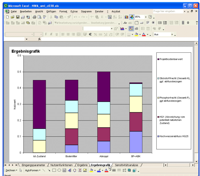
Abbildung 68: Excel-Bewertungstool – Ergebnisgrafik
