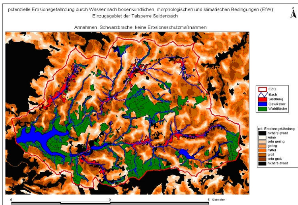
Abbildung 97: Potenzielle Erosionsgefährdung (EfW) im Einzugsgebiet der TS Saidenbach (Annahmen: Schwarzbrache, keine Erosionsschutzmaßnahmen)
