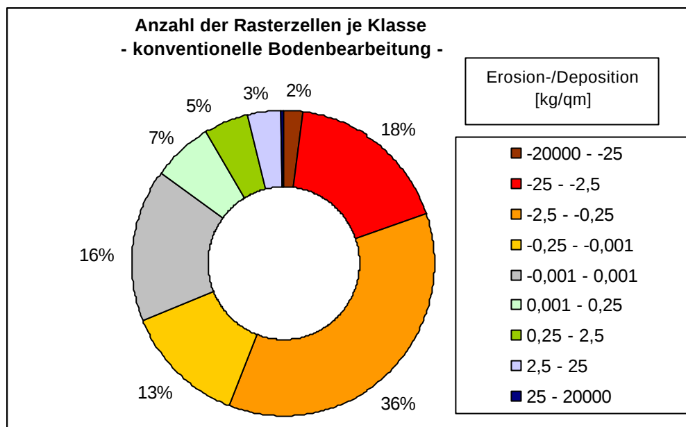
Abbildung 100: Prozentuale Verteilung der Rasterzellen (10*10m) der verschiedenen Erosions- sowie Depositionsklassen bei EROSION 3D-Simulation eines „worstcase“-Szenarios im Teil-einzugsgebiet „Kunstteich“ bei Annahme einer flächendeckend konventionellen Bodenbearbeitung (20jährlicher Niederschlag)
