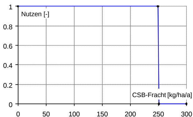
Abbildung 17: Nutzenfunktion (Beispiel 1)
