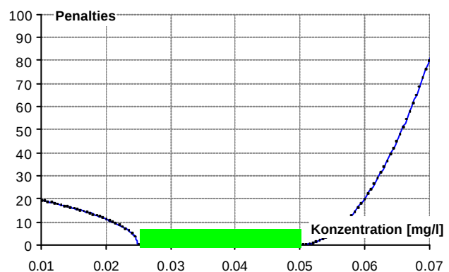
Abbildung 21: Penaltyfunktion (Beispiel 2)
