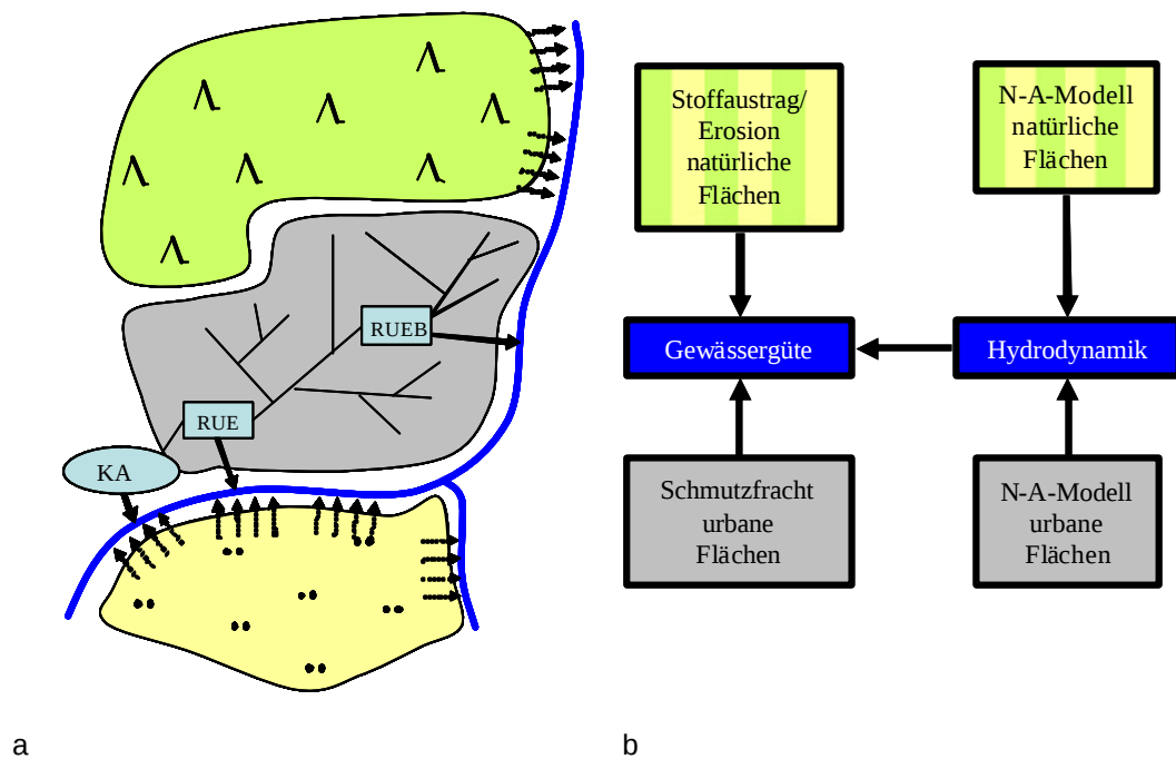
Abbildung 126: Systemgrenzen Modellsystem
