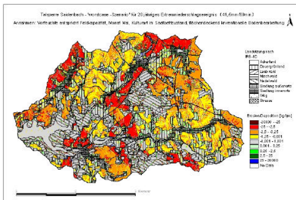
Abbildung 98: Worstcase“-Szenario für ein 20jähriges Extremniederschlagsereignis für das Einzugsgebiet der Talsperre Saidenbach (Simulation mit EROSION 3D)
