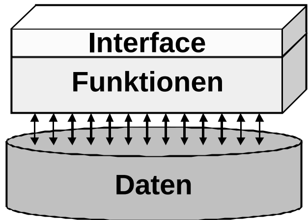
Abbildung 31: DSS-Aufbau (2)
