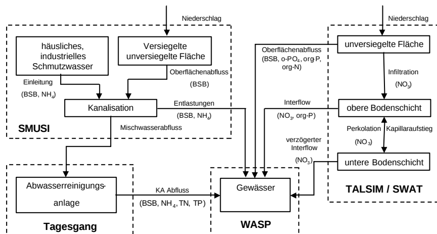
Abbildung 127: Modellsystem
