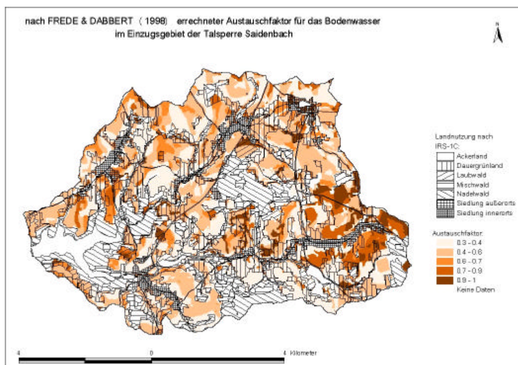
Abbildung 108: Errechneter Austauschfaktor für das Bodenwasser nach FREDE & DABBERT (1998) für das Einzugsgebiet Talsperre Saidenbach
