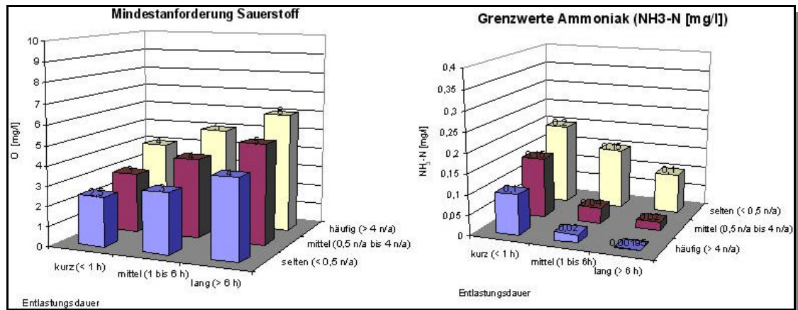
Abbildung 13: Komplexe Zielvariable „9er-Matrix“
