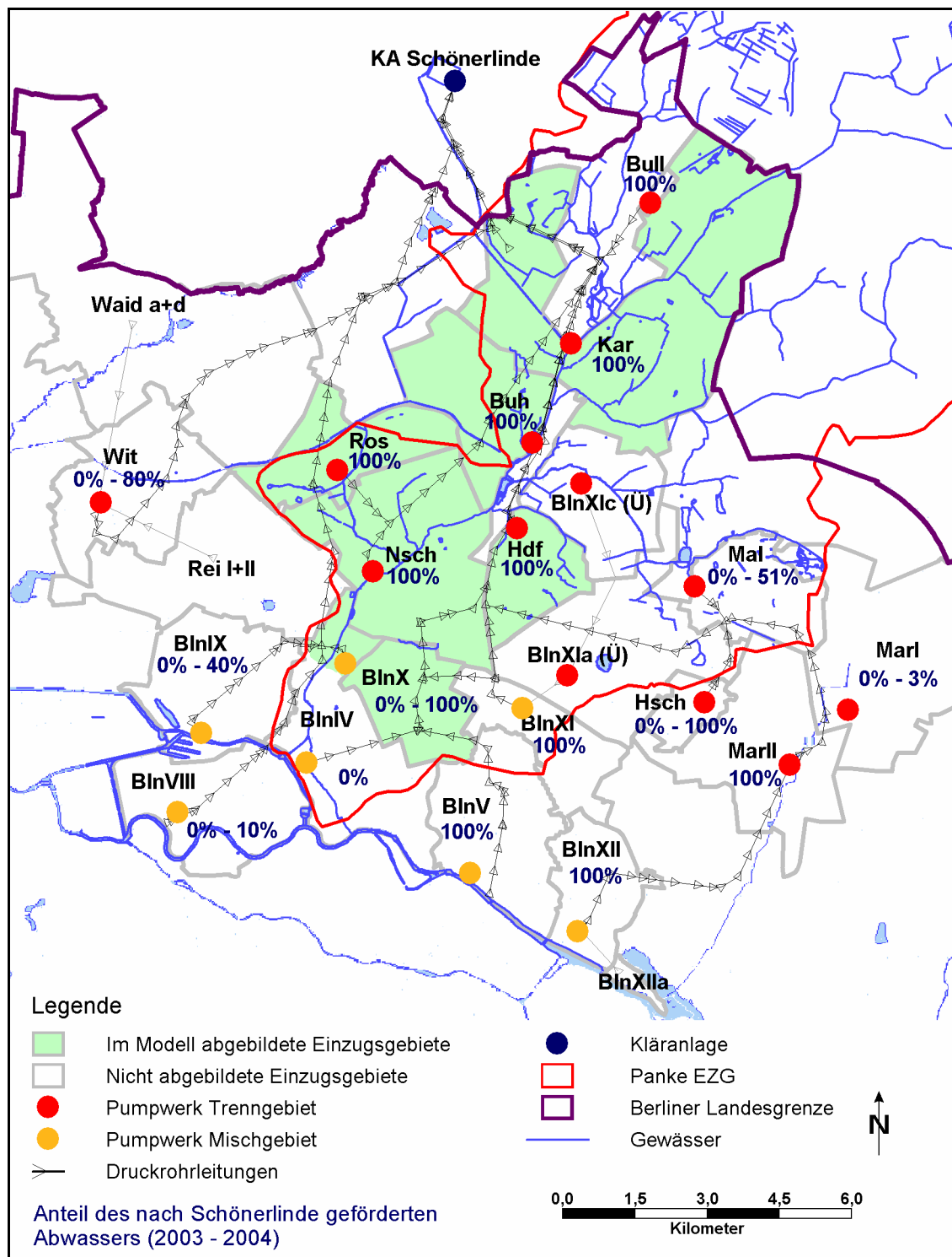
Abbildung 79: Einzugsgebiete der KA Schönerlinde
