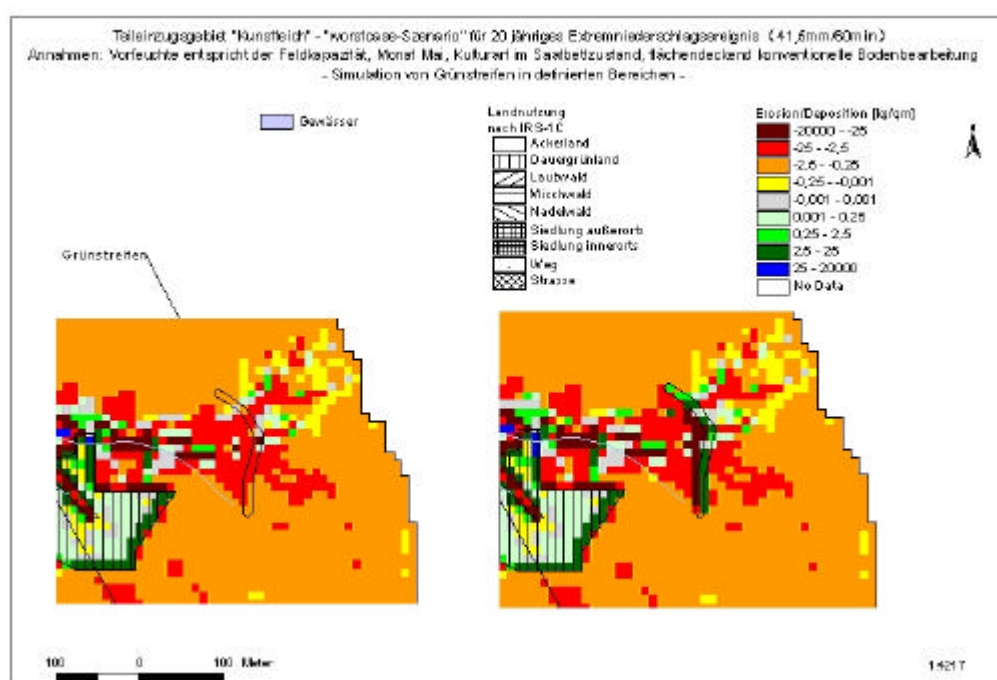
Abbildung 103: Bodenerosion durch Wasser ohne (linkes Bild) und mit Anlage eines Grünstreifen (rechtes Bild) im Teileinzugsgebiet „Kunstteich“ (Modellierung mit EROSION 3D)
