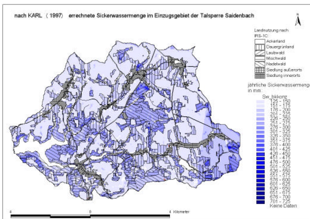
Abbildung 107: Errechnete Sickerwassermenge nach KARL (1997) im Einzugsgebiet der Talsperre Saidenbach
