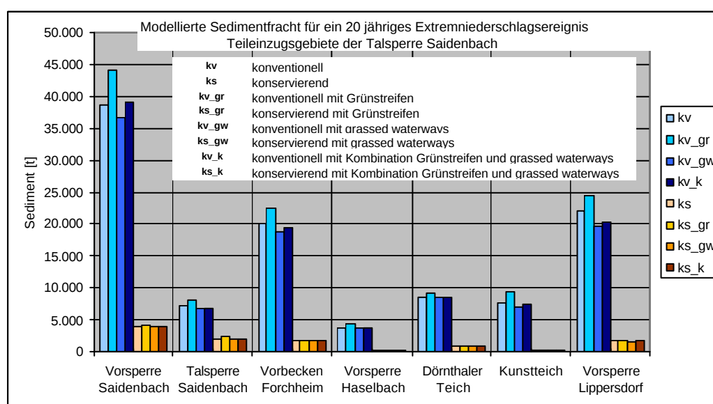
Abbildung 104: Modellierte Sedimentfracht für ein 20-jähriges Extremniederschlagsereignis für unterschiedliche Szenarien in den Teileinzugsgebieten der Talsperre Saidenbach
