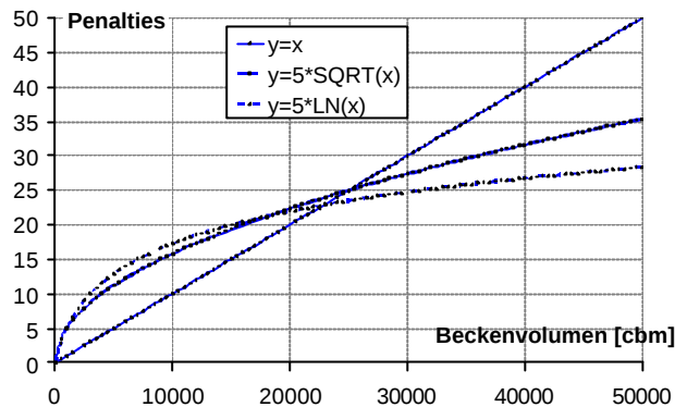
Abbildung 22: Penaltyfunktionen (Beispiel 3)
