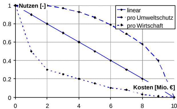
Abbildung 19: Nutzenfunktion (Beispiel 3)
