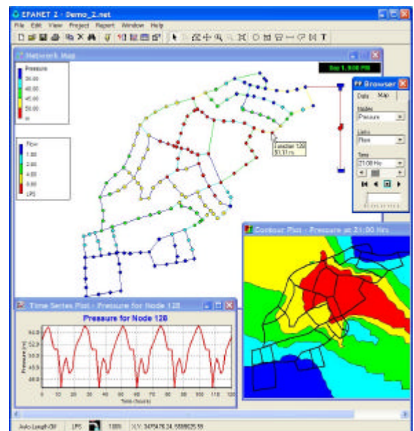
Abbildung 36: DSSF-Komponente Modelle
