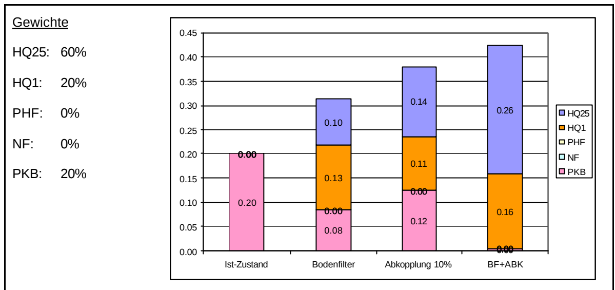
Abbildung 29: Beispiel - Gewichtung 2
