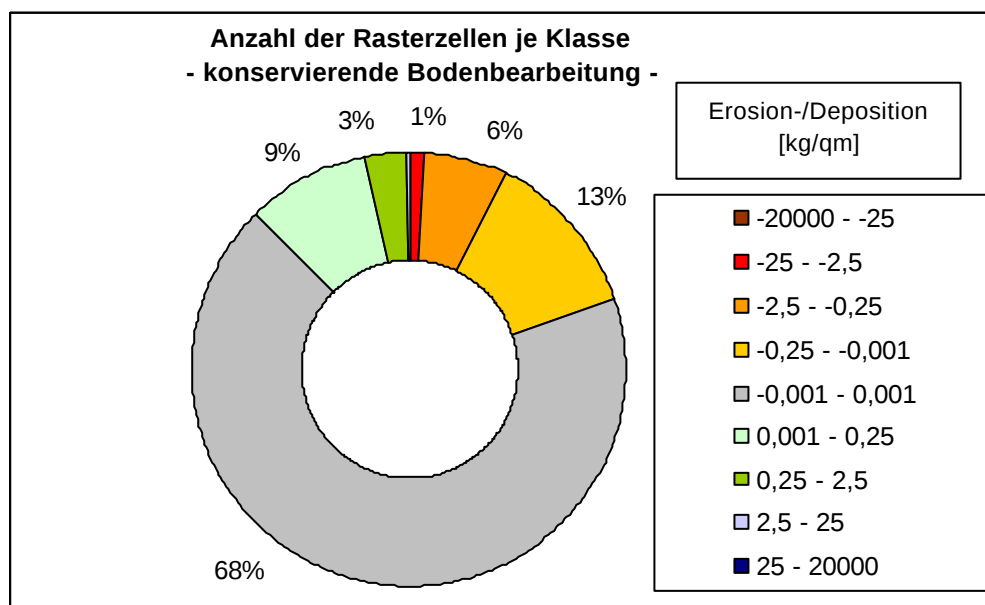
Abbildung 101: Prozentuale Verteilung der Rasterzellen (10*10m) der verschiedenen Erosions- sowie Depositionsklassen bei EROSION 3D-Simulation eines „bestcase“-Szenarios im Teil-einzugsgebiet „Kunstteich“ bei Annahme einer flächendeckend konservierenden Bodenbearbeitung (20jährlicher Niederschlag)
