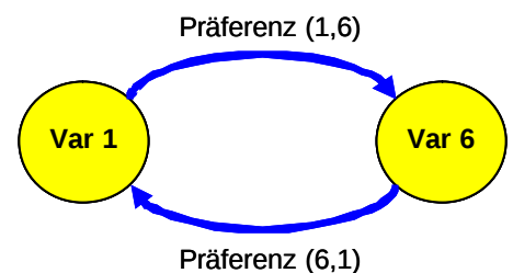
Abbildung 24: PROMETHEE- Prinzip des Präferenzindex
