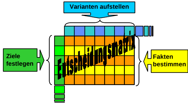
Abbildung 32: DSSF-Komponente Entscheidungsmatrix
