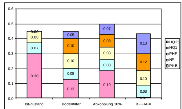
Abbildung 37: DSSF-Komponente Bewertung
