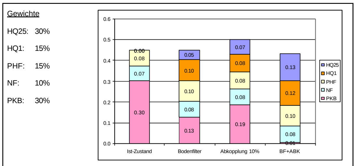
Abbildung 28: Beispiel - Gewichtung 1
