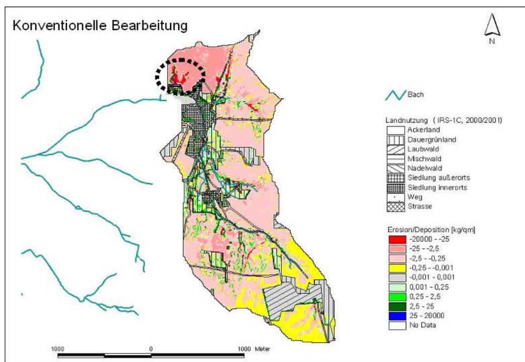
Abbildung 102: Simulation eines worstcase-Szenarios mit EROSION 3D im Teileinzugsgebiet „Kunsteich“ bei Annahme einer flächendeckend konventionellen Bodenbearbeitung (20jähriger Niederschlag; Bereich linienhafter Erosion siehe gestrichelte Umrandung)
