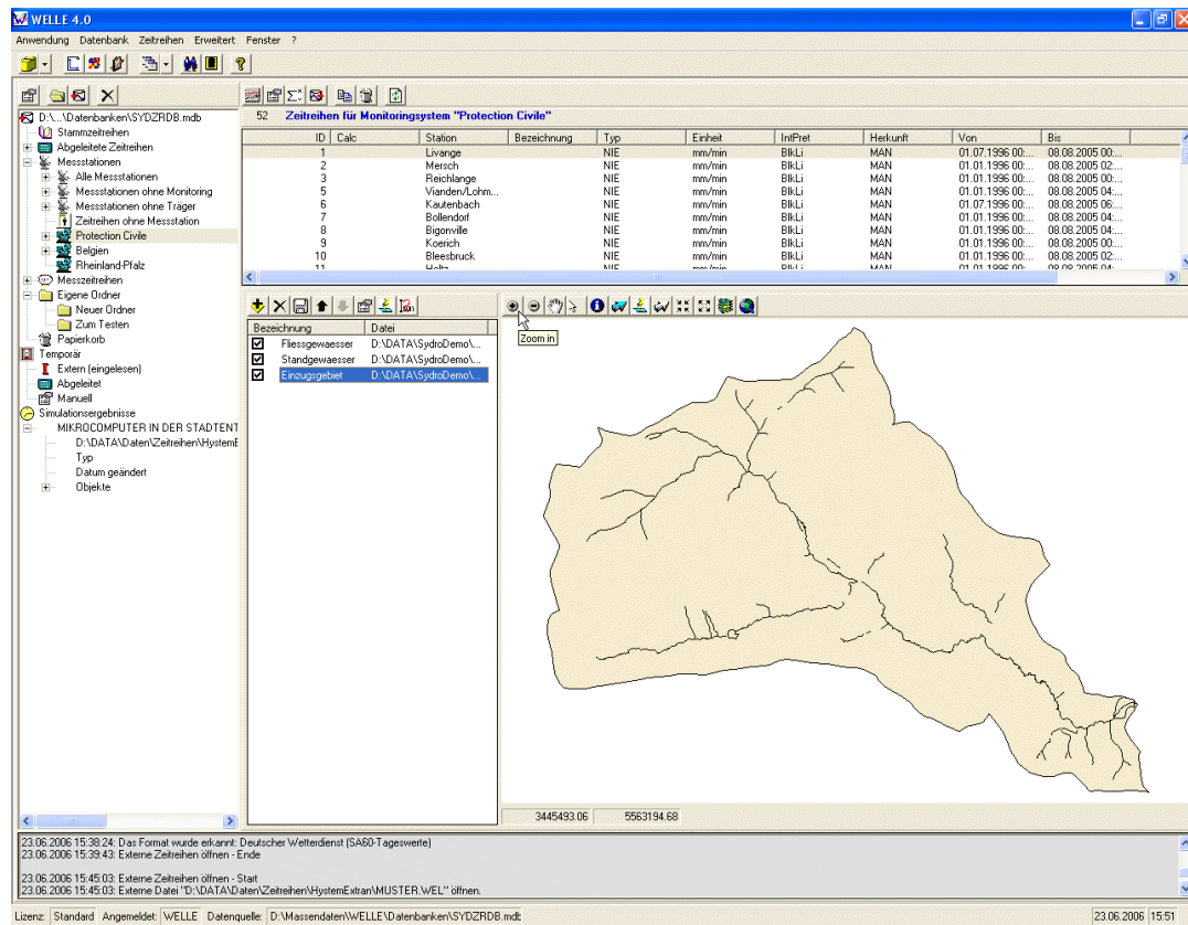
Abbildung 63: WELLE-Explorer mit Kartendarstellung
