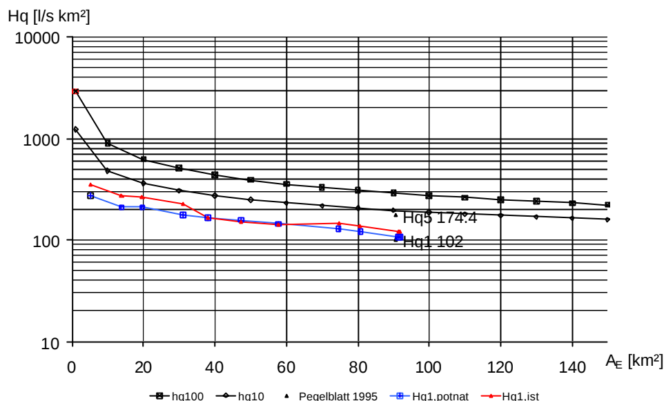
Abbildung 125: Hochwasserabflussspenden Modaugebiet
