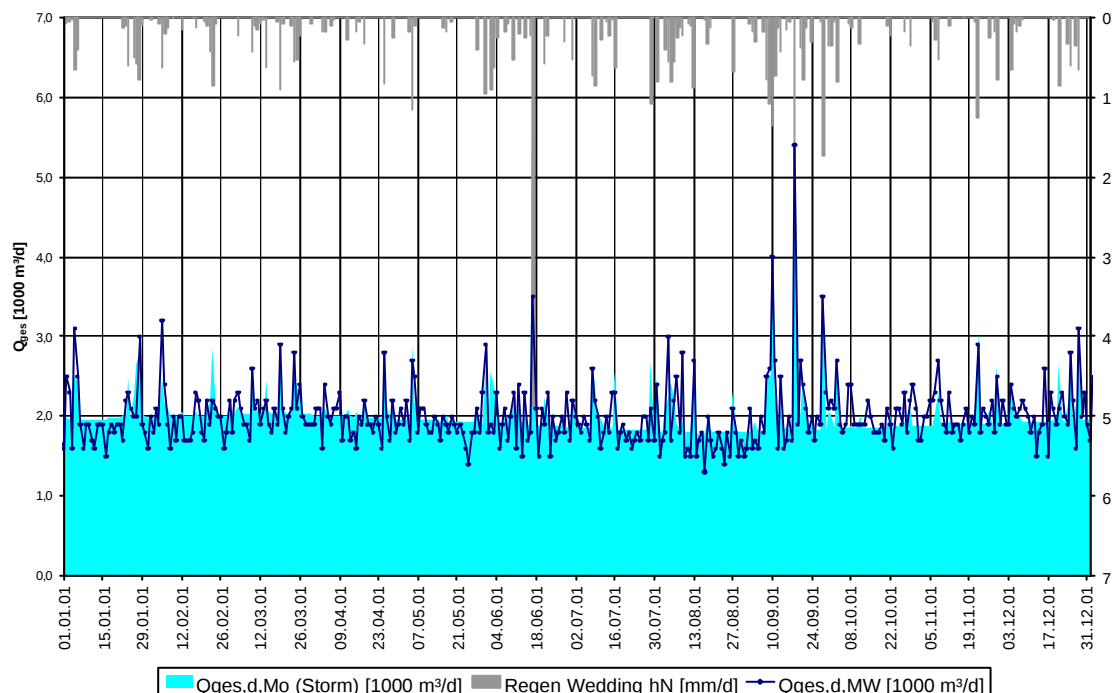
Abbildung 81: Vergleich der Pumpwerksfördermengen mit den Ergebnissen der Kalibrierung des STORM Modells (exemplarisch für das Pumpwerk Rosenthal und das Jahr 2001)
