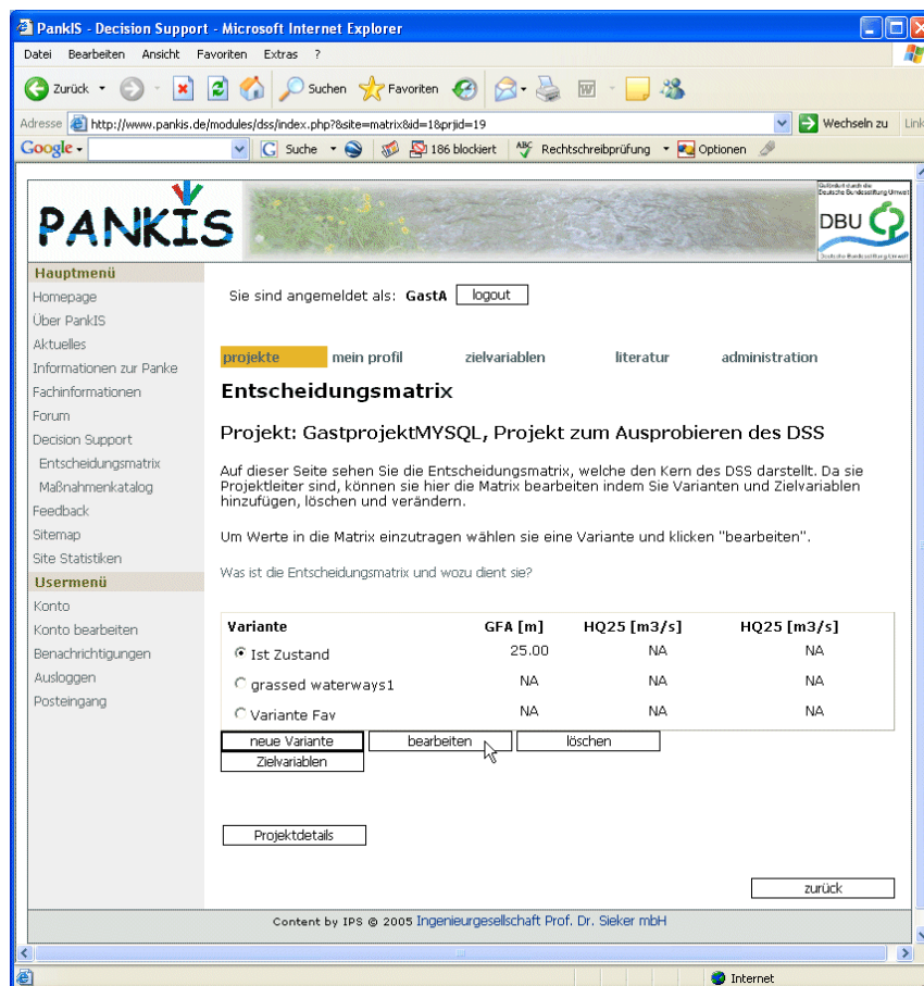
Abbildung 40: DSSF-Anwendung „Entscheidungsmatrix aufstellen – webbasiert“
