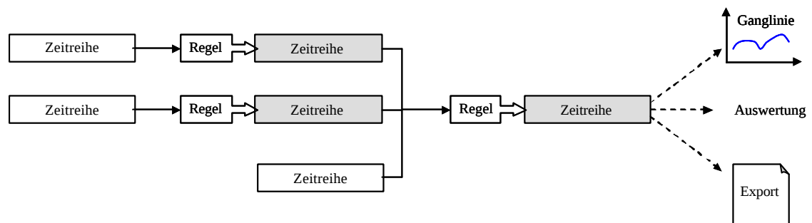
Abbildung 56: WELLE-Zeitreihen ableiten (rekursiv)
