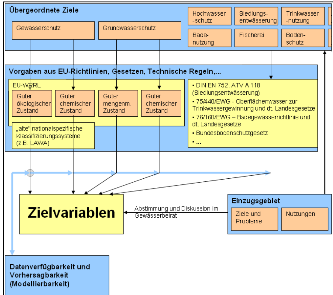
Abbildung 12: Von Zielen zu Zielvariablen
