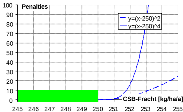
Abbildung 20: Penaltyfunktion (Beispiel 1)
