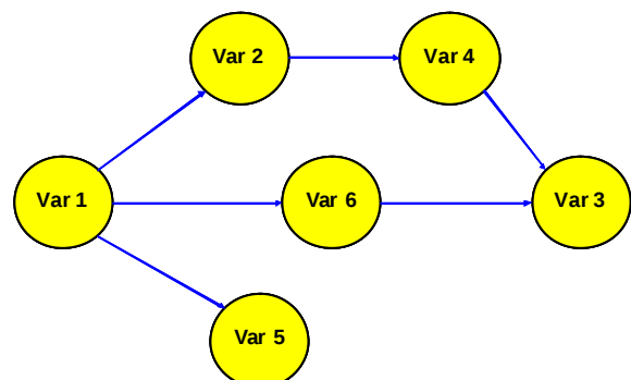
Abbildung 25: PROMETHEE- Muster einer partiellen Präordnung
