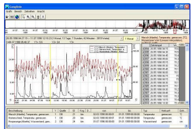
Abbildung 34: DSSF-Komponente Zeitreihenmanagement
