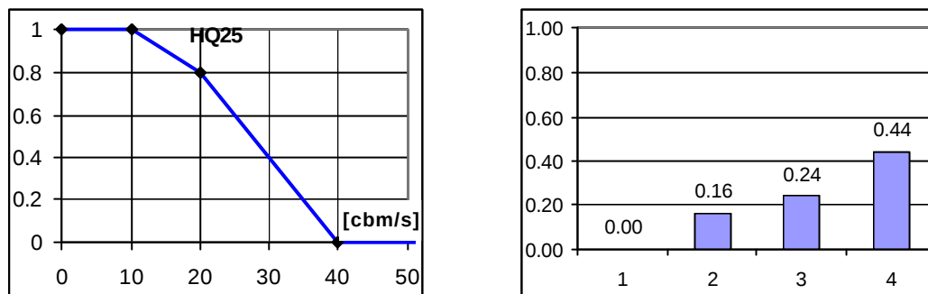
Abbildung 26: Beispiel – Nutzenfunktion und Nutzwerte für die Zielvariable HQ_{25}
