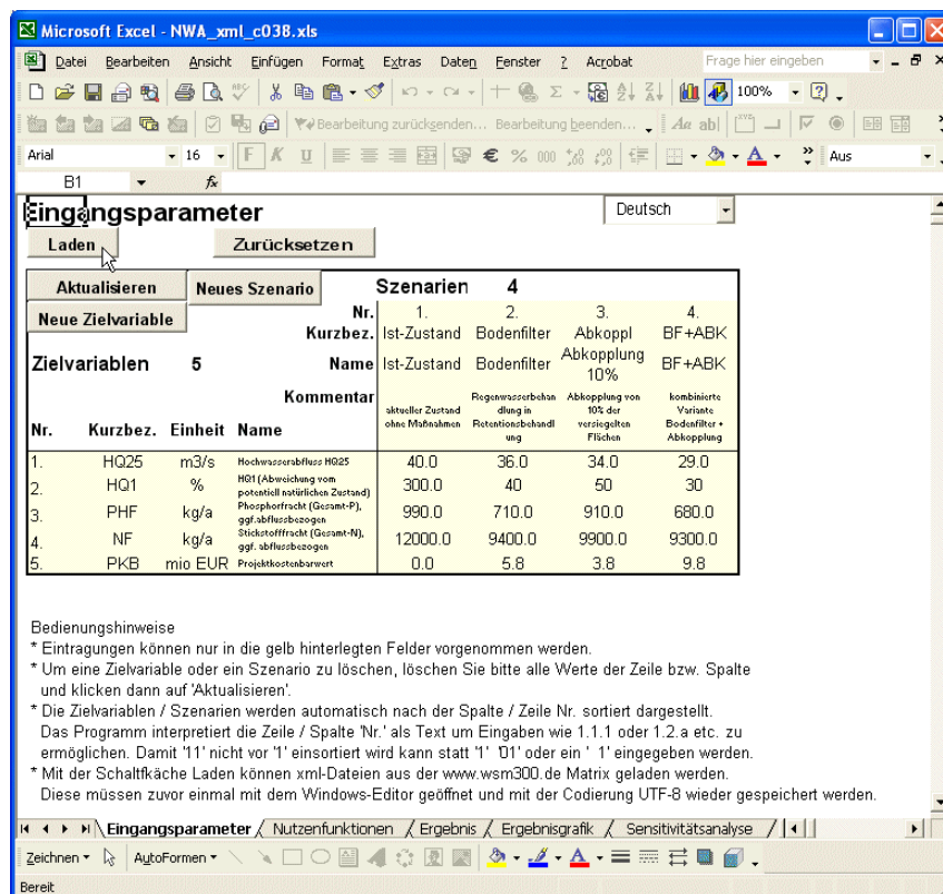
Abbildung 65: Excel-Bewertungstool – Eingangsparameter
