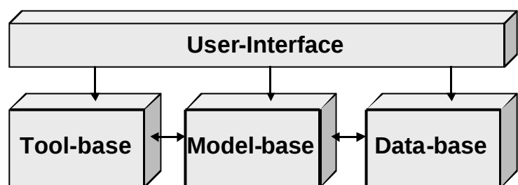
Abbildung 30: DSS-Aufbau (1)
