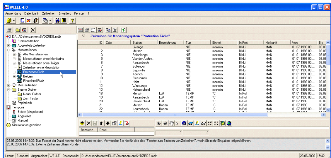
Abbildung 51: WELLE-Explorer
