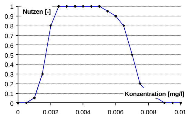
Abbildung 18: Nutzenfunktion (Beispiel 2)
