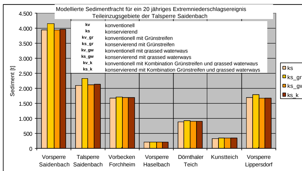
Abbildung 105: Modellierter Sedimentfracht für ein 20-jähriges Extremniederschlagsereignis für unterschiedliche Szenarien in den Teileinzugsgebieten der Talsperre Saidenbach. Detaildarstellung für konservierende Bodenbearbeitung mit ergänzenden Schutzmaßnahmen (grassed waterways, Grünstreifen usw., Gesamtdarstellung der Szenarien s. Abbildung 104)
