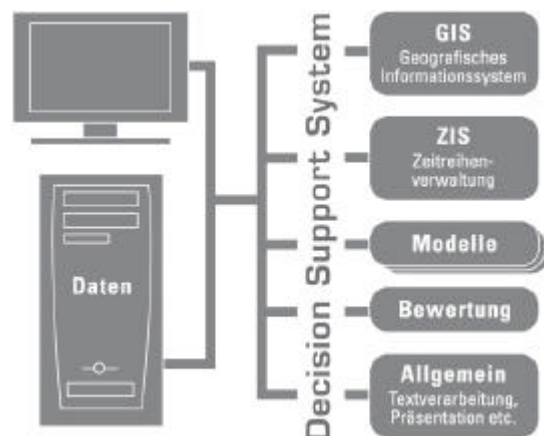
Abbildung 38: DSSF-Komponenten
