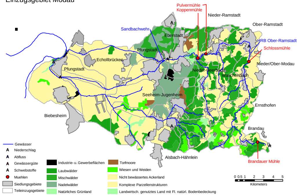
Abbildung 120: Nutzungen im Modaugebiet
