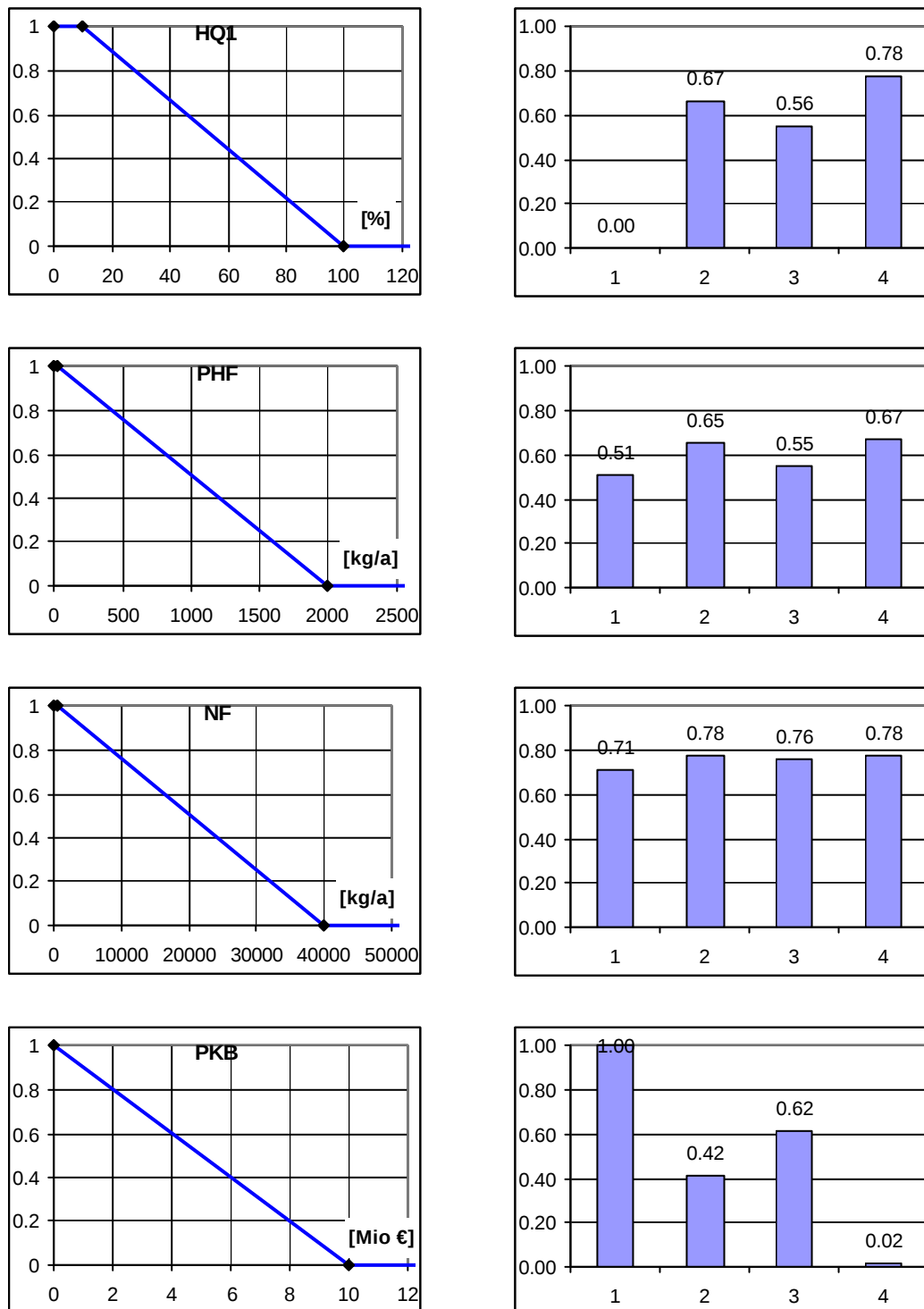
Abbildung 27: Beispiel – Nutzenfunktion und Nutzwerte für die Zielvariable PKB
