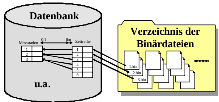
Abbildung 50: WELLE-Datenhaltung
