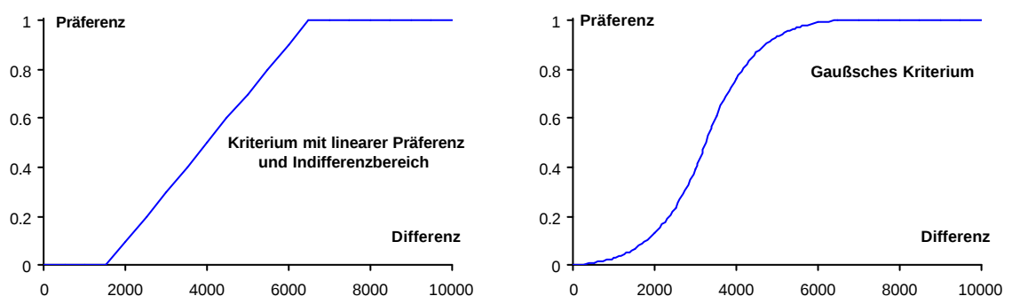
Abbildung 23: Beispiele für Präferenzfunktionen
