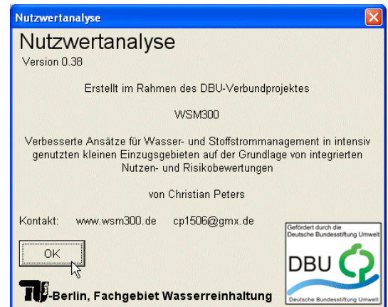
Abbildung 64: Excel-Bewertungstool
