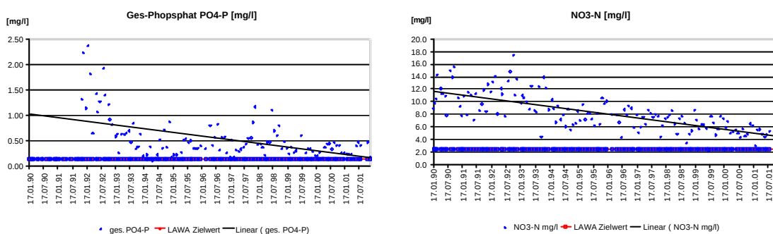
Abbildung 123: Nährstoffkonzentrationen Messstelle Stockstadt
