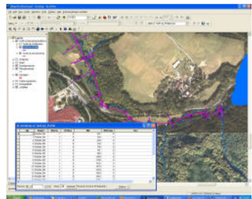
Abbildung 33: DSSF-Komponente GIS
