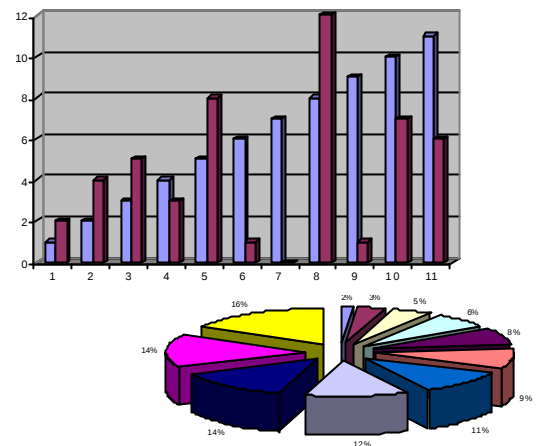
Abbildung 35: DSSF-Komponente Statistik
