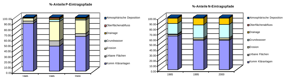
Abbildung 122: Prozentuale Anteile der Eintragspfade von Phosphor und Stickstoff
