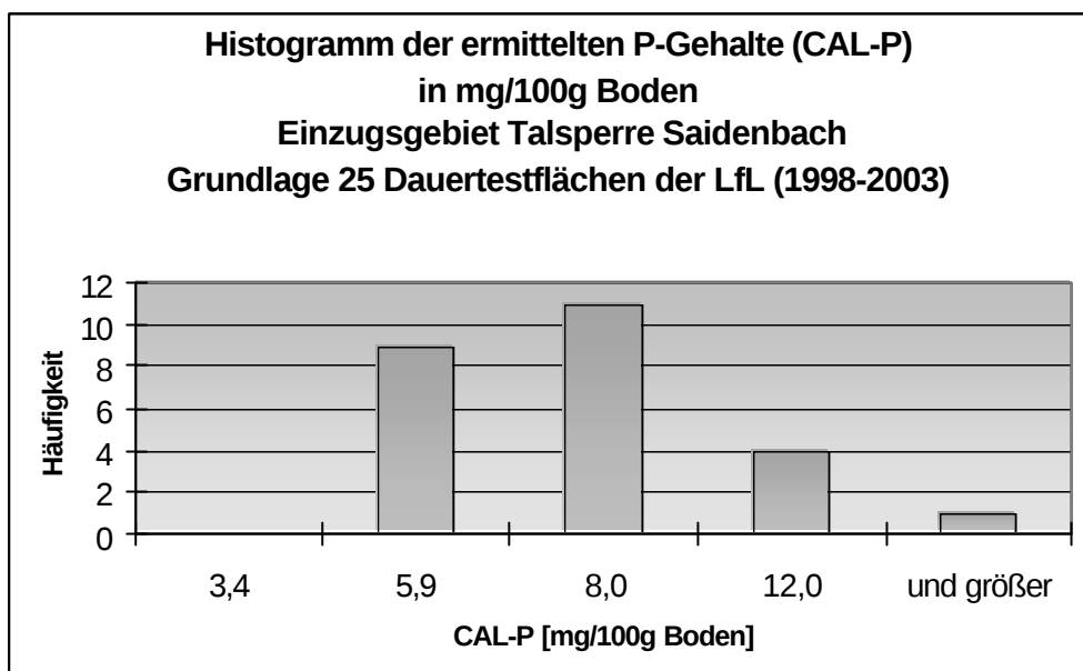
Abbildung 106: Häufigkeitsverteilung nach Nährstoffversorgungsstufen der ermittelten CAL-P-Gehalte der Dauertestflächen der LfL im Einzugsgebiet Talsperre Saidenbach
