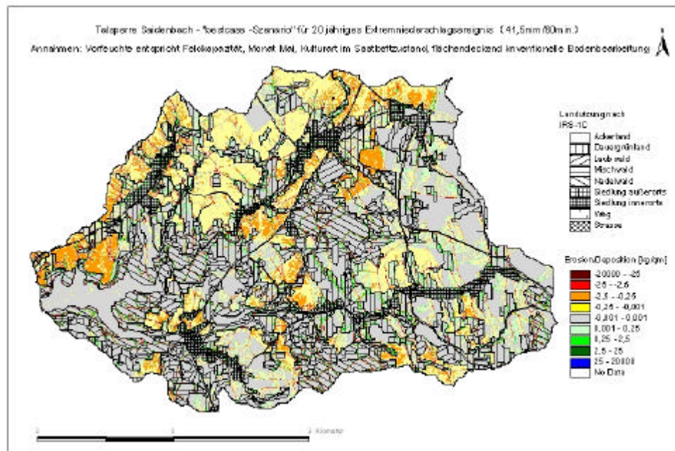
Abbildung 99: „Bestcase“-Szenario für ein 20jähriges Extremniederschlagsereignis für das Einzugsgebiet der Talsperre Saidenbach (Simulation mit EROSION 3D)
