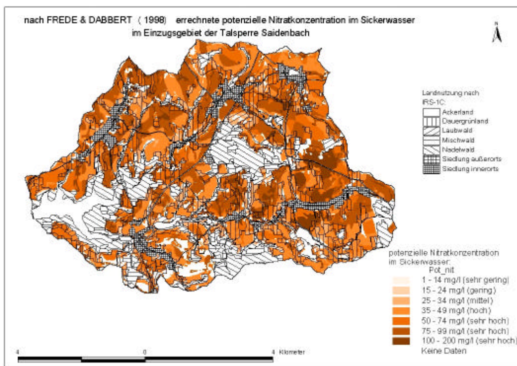
Abbildung 109: Errechnete potenzielle Nitratkonzentration im Sickerwasser nach FREDE & DABBERT (1998)
