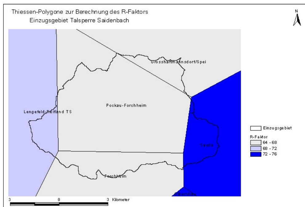
Abbildung 96: Thiessen-Polygone zur Berechnung des R-Faktor
