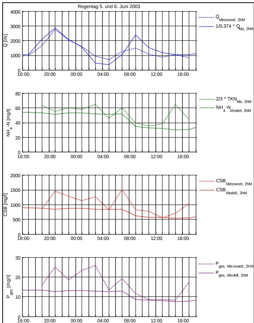
Abbildung 85: Vergleich des Ablaufs des ADL-Modells mit Zulaufsmesswerten der Kläranlage 2h-Mittelwerte 05. und 06.06.2003
