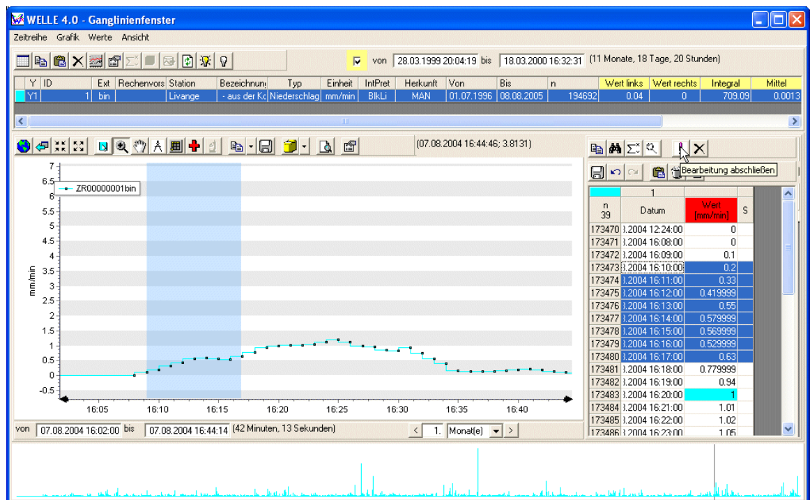
Abbildung 55: WELLE-Ganglinienfenster mit Punktdarstellung im Bearbeitungsmodus
