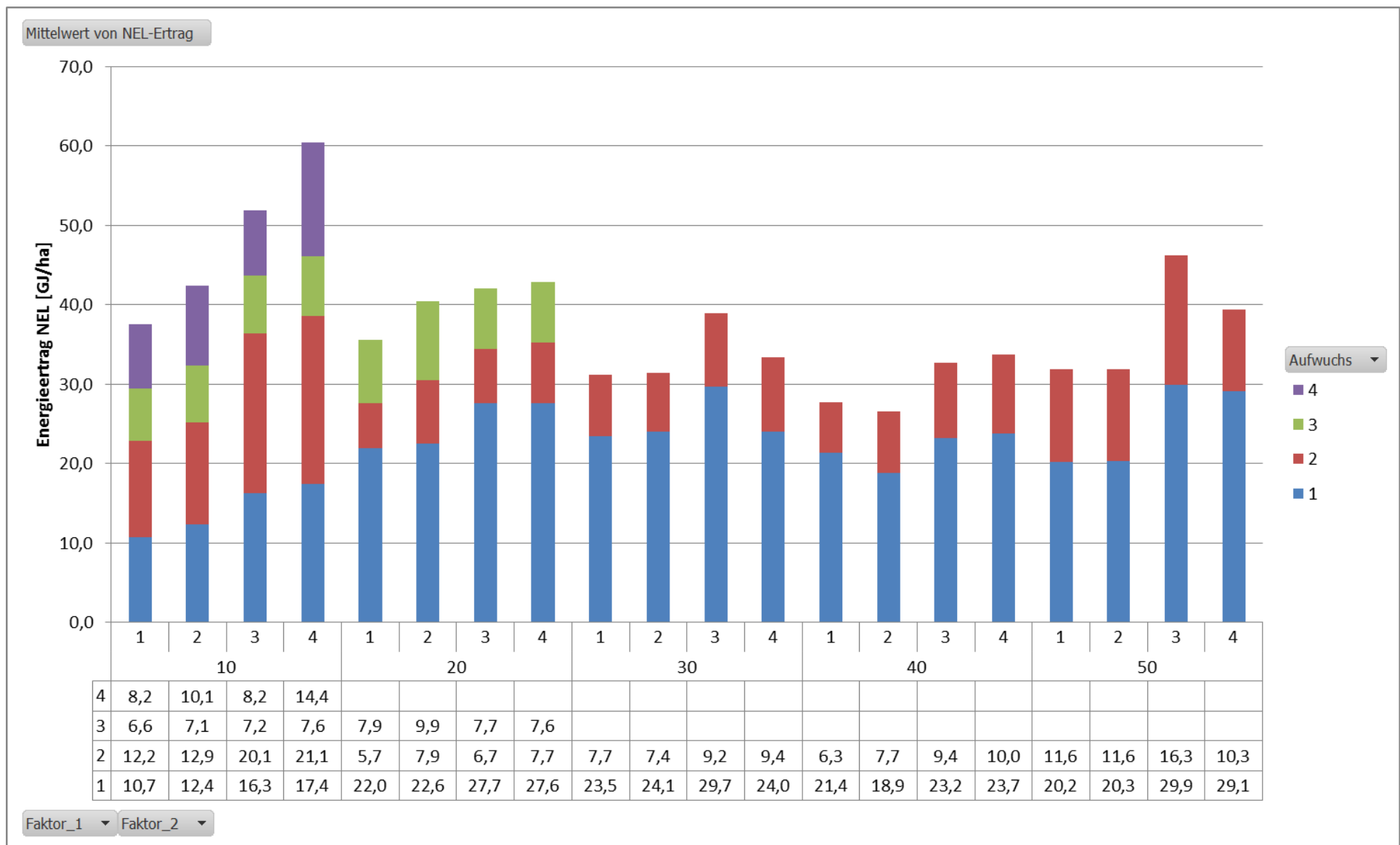
Abbildung 2: Versuchsergebnisse 032: Energieertrag der Versuchsvarianten im Jahr 2014.
