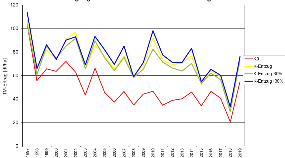
Entwicklung der Trockenmasseerträge der Varianten mit unterschiedlicher K-Düngung in den Jahren 1997 bis 2019 in Christgrün
