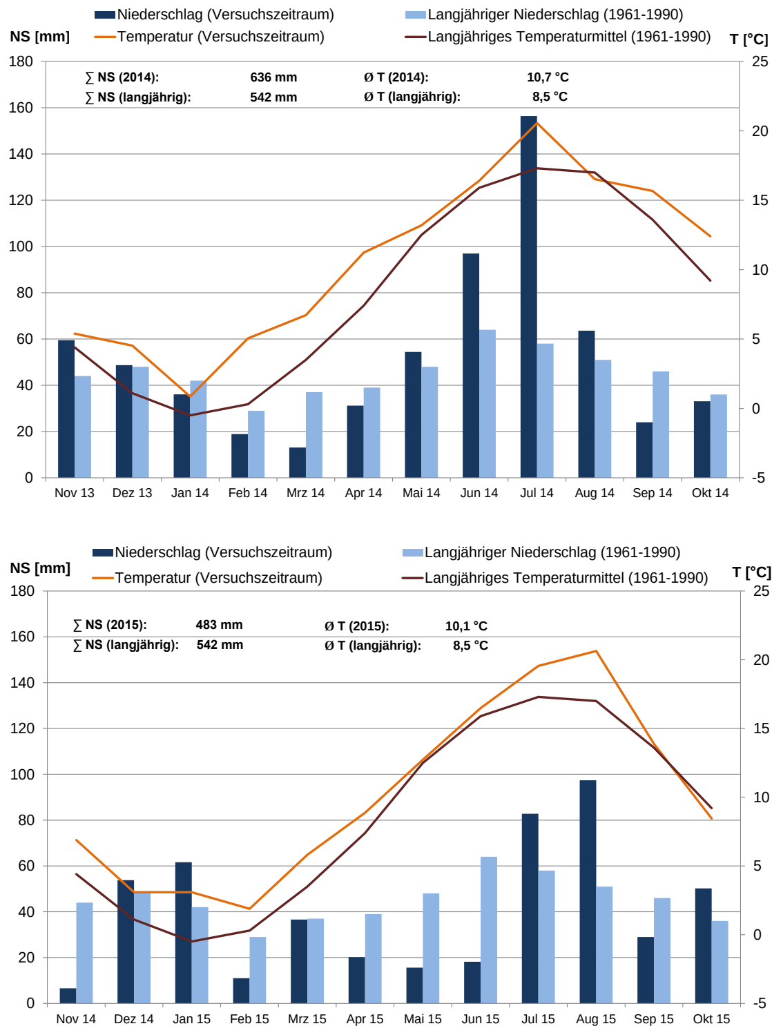
Abbildung 67: Witterungsverlauf am Standort Lückstedt in den Versuchsjahren 2014 und 2015.
