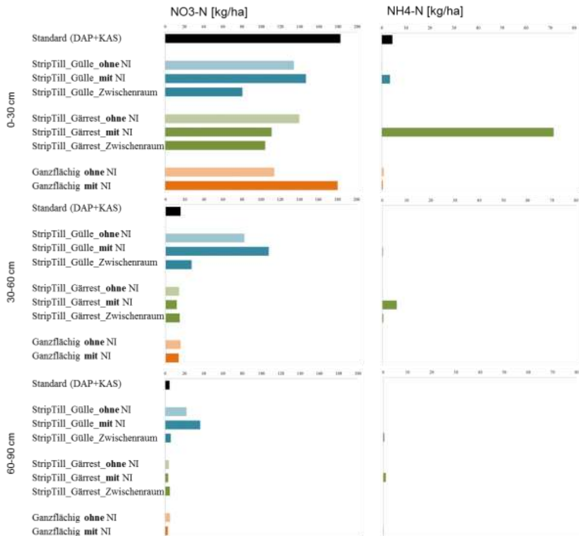
Abbildung 79: NO 3 -N und NH 4 -N-Werte in kg/ha im 5 Blattstadium; Lüttewitz 23.06.2014.
