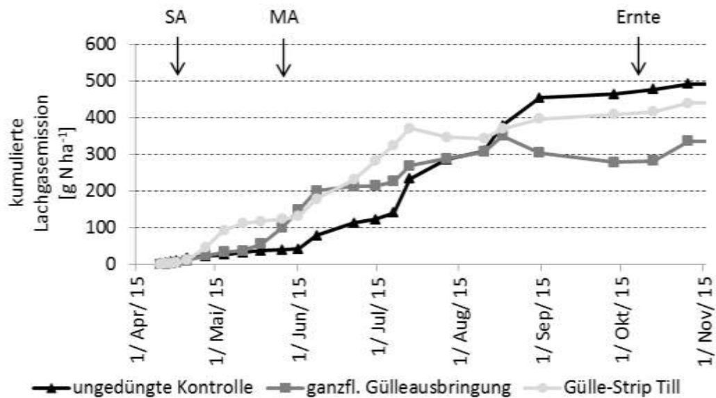
Abbildung 40: Kumulierter Verlauf der Lachgasflüsse in der Reihe im Zeitraum April bis November 2015 am Standort Kossebau; SA = Gülleausbringung, MA= mineralische Düngung.
