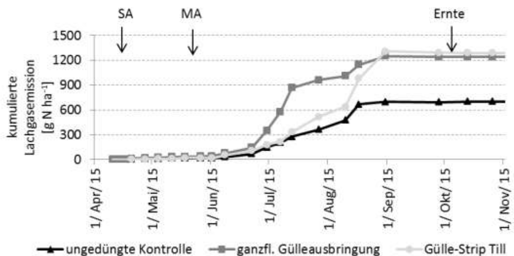
Abbildung 41: Kumulierter Verlauf der Lachgasflüsse in der Zwischenreihe im Zeitraum April bis November 2015 am Standort Kossebau; SA = Gülleausbringung, MA= mineralische Düngung.
