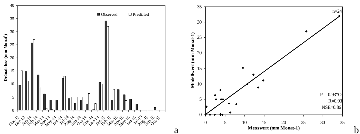
Abbildung 24: a) Reale und modellierte monatliche Dränabflussmengen, b) Regressionsanalysen zwischen den realen und modellierten Dränabflussmengen.
