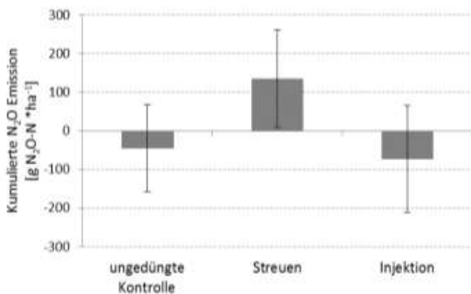
Abbildung 56: Kumulierte Lachgasemission von März 2014 bis zur Ernte im August 2014 am Standort Nossen. Die Fehlerbalken entsprechen der Standardabweichung (n=4).
