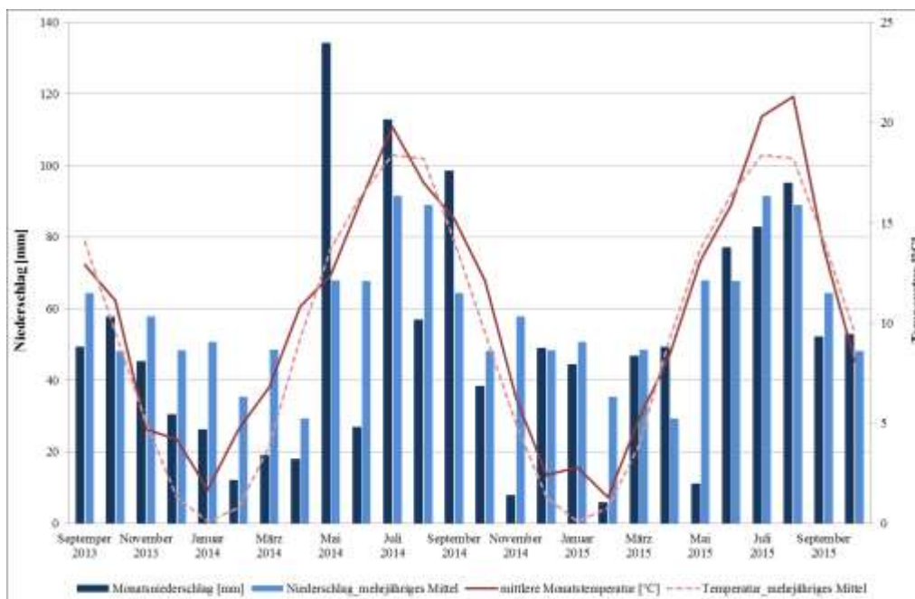
Abbildung 17: Mittlere Monatstemperaturen und Monatsniederschläge sowie langjähriges Mittel der Station Nossen, 2013-2015.
