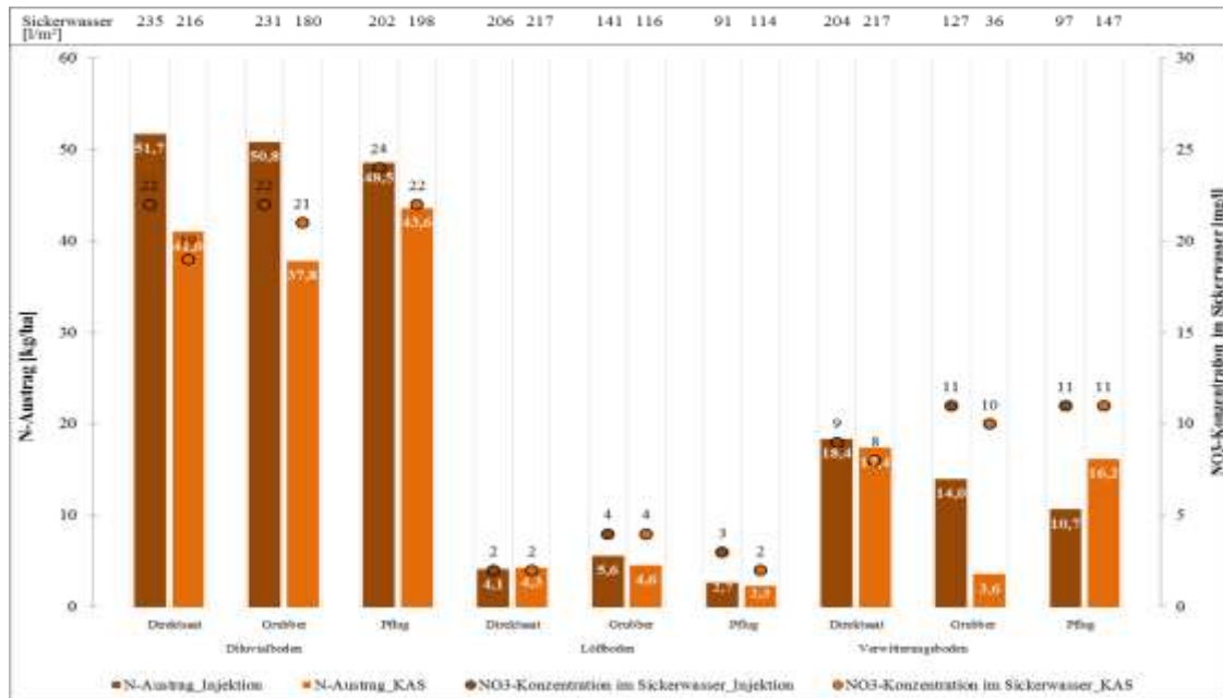
Abbildung 109: Einfluss von Bodenart, Bodenbearbeitung und Düngeform auf Sickerwassermenge und NO 3 -Konzentration im Sickerwasser und N-Austrag; Nossen 2015
