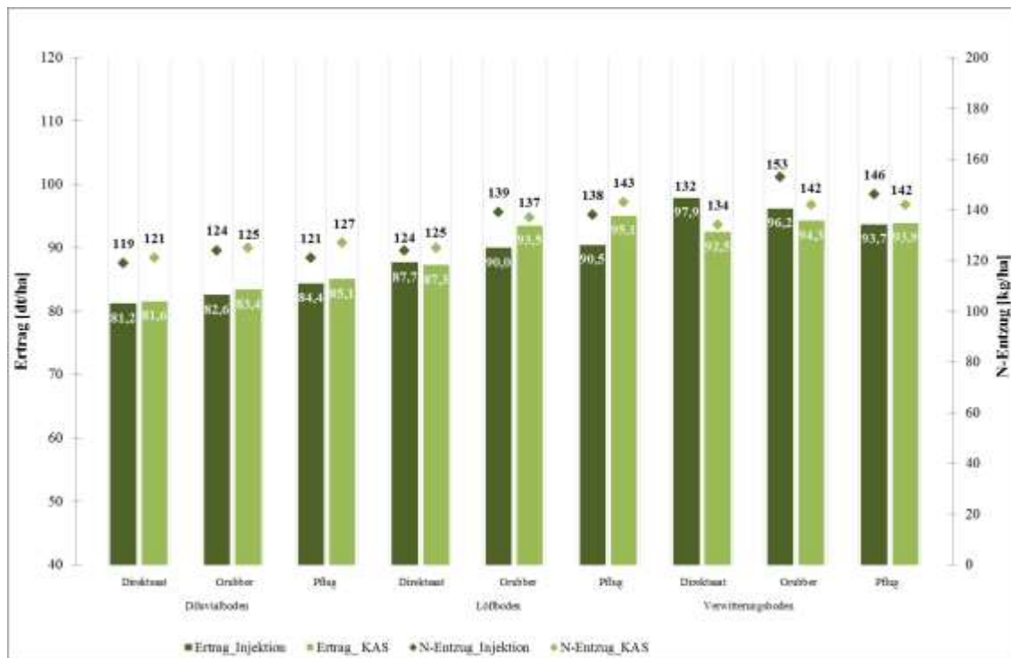
Abbildung 106: Wirkung der Düngevarianten auf Weizenерtrag und N-Entzug bei unterschiedlicher Bodenbearbeitung auf den Standorten D, Löß und V; Nossen 2014
