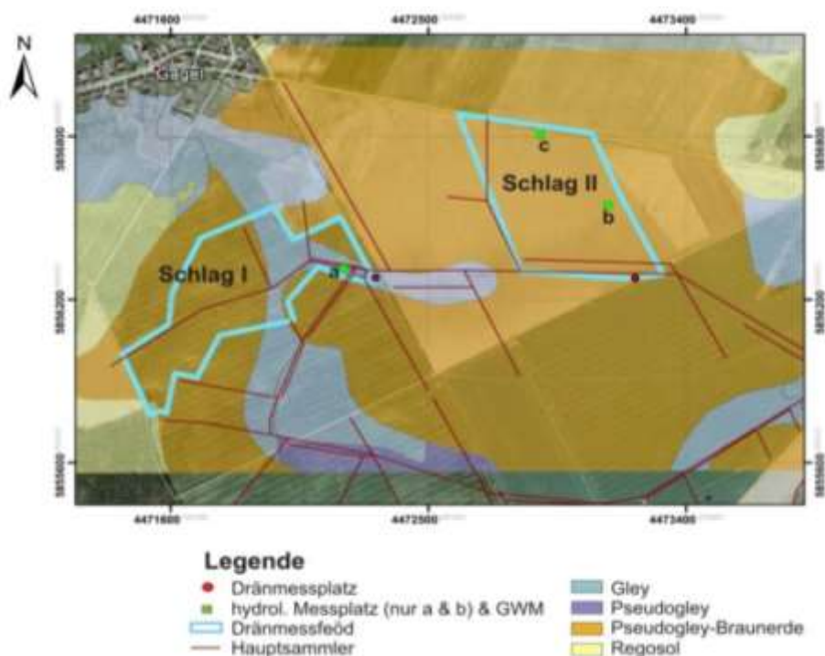
Abbildung 1: Untersuchungsgebiet Lückstedt.
