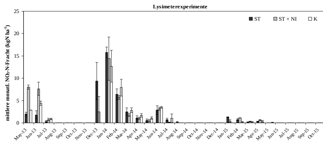
Abbildung 22: Gegenüberstellung der Lysimetervarianten ST, ST+NI und K hinsichtlich a) mittlerer monatlicher Sickerwassermenge; mittlerer monatlicher \text{NO}_3\text{-N} -Konzentration im Sickerwasser; c) mittlerer monatlicher \text{NO}_3\text{-N} -Fracht.
