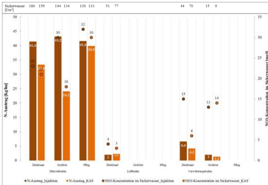
Abbildung 108: Einfluss von Bodenart, Bodenbearbeitung und Düngeform auf Sickerwassermenge und NO 3 -Konzentration im Sickerwasser und N-Austrag; Nossen 2014
