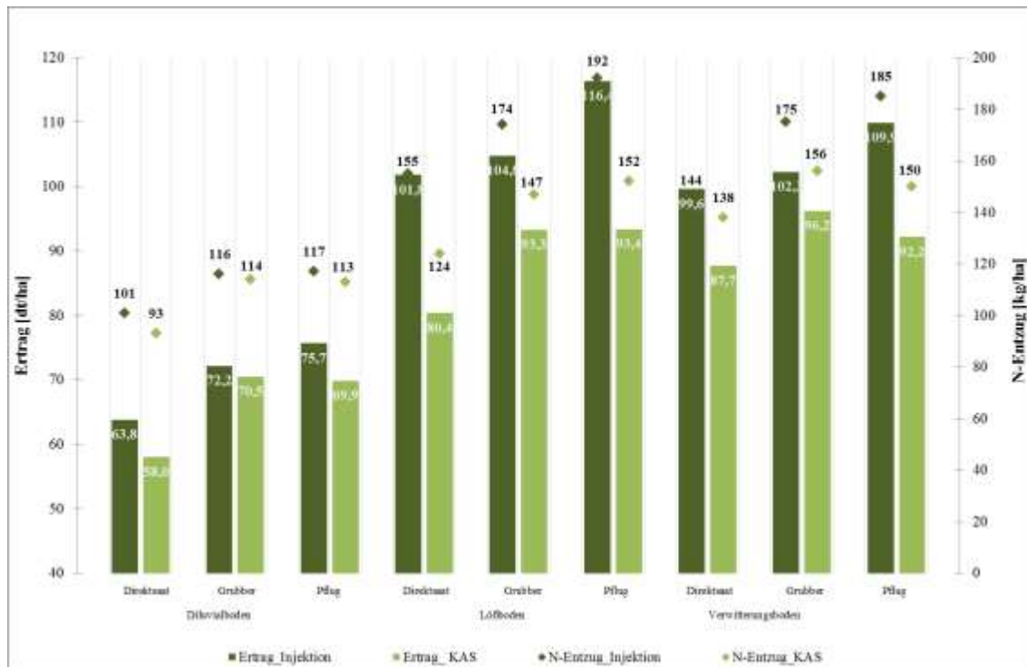
Abbildung 107: Wirkung der Düngevarianten auf den Gerstenenertrag und N-Entzug bei unterschiedlicher Bodenbearbeitung auf den Standorten D, Lö und V; Nossen 2015
