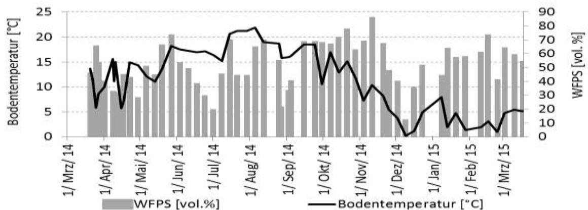
Abbildung 60: Verlauf der Bodentemperatur [°C] und WFPS [vol. %] am Standort Nossen von März 2014 bis März 2015 über alle Varianten gemittelt.
